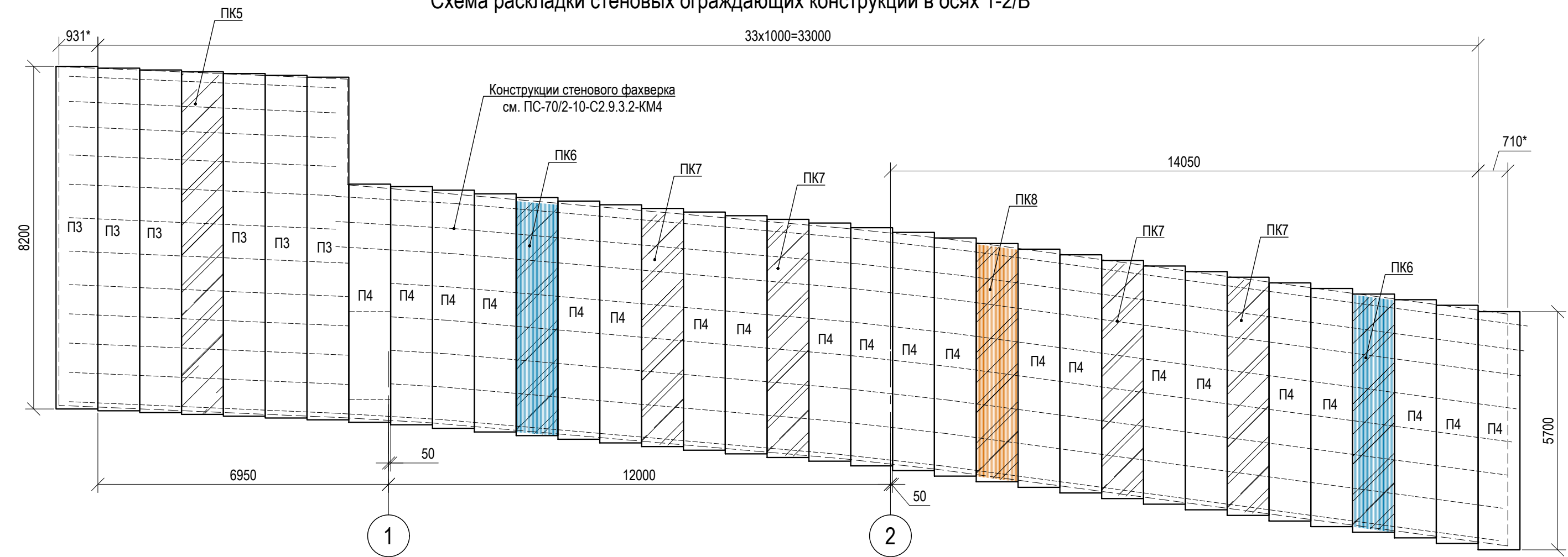
Схема раскладки стеновых ограждающих конструкций в осях 1-2/В
