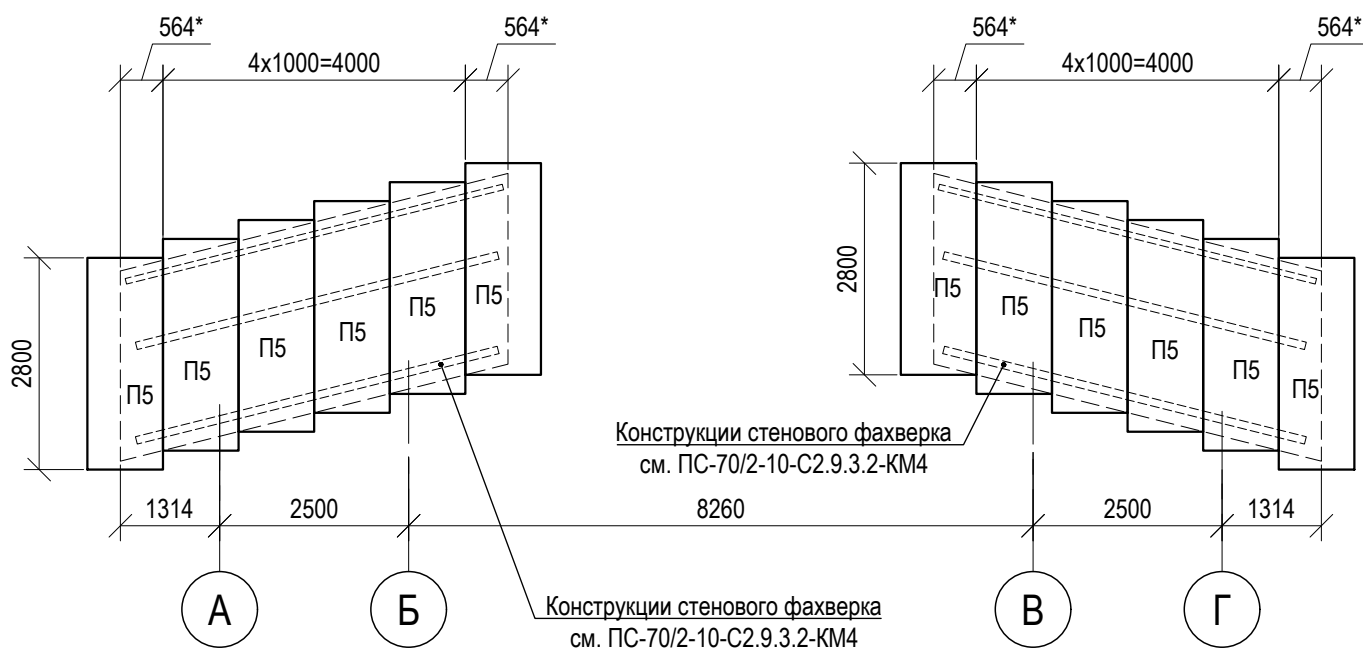
Схема раскладки стеновых ограждающих конструкций в осях А-Г/1
