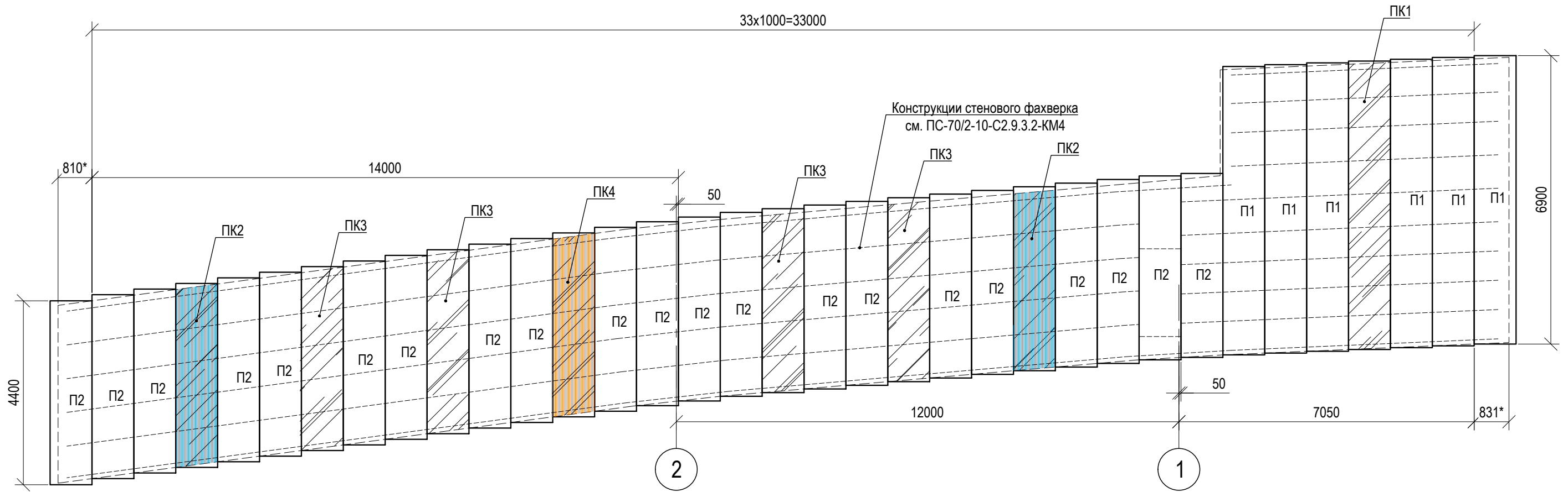
Схема раскладки стеновых ограждающих конструкций в осях 2-1/Г
