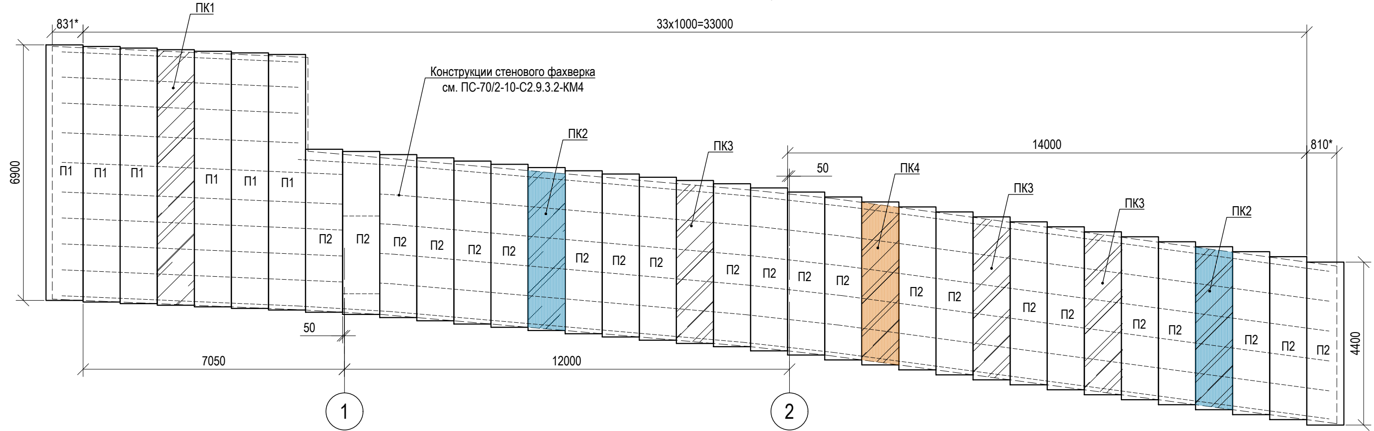
Схема раскладки стеновых ограждающих конструкций в осях 1-2/А
