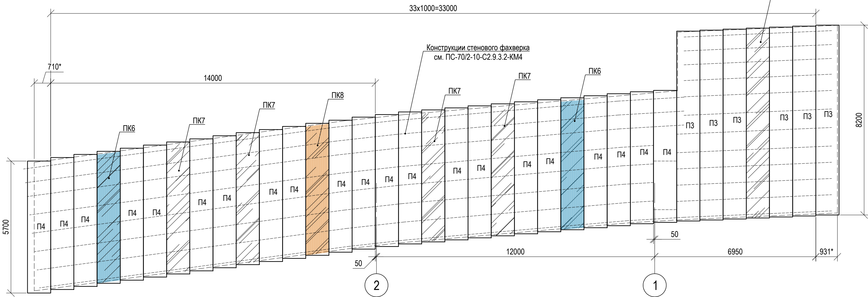
Схема раскладки стеновых ограждающих конструкций в осях 2-1/Б
